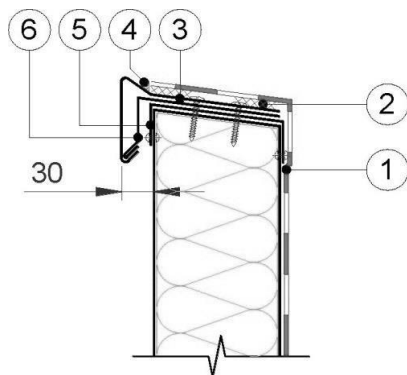
Рис. 28 Примыкание к парапетной стене высотой менее 500 мм с использованием отлива
