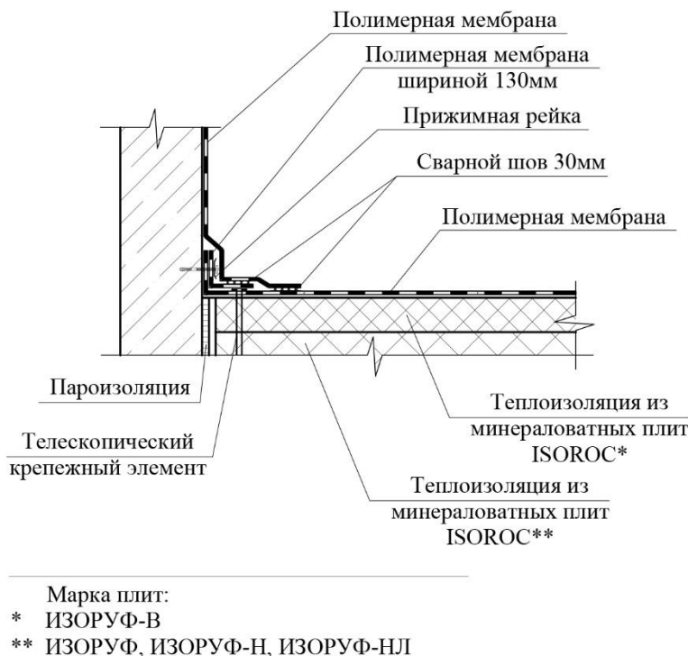
Рис. 20 Устройство кровельного гидроизоляционного материала на переходном бортике.
