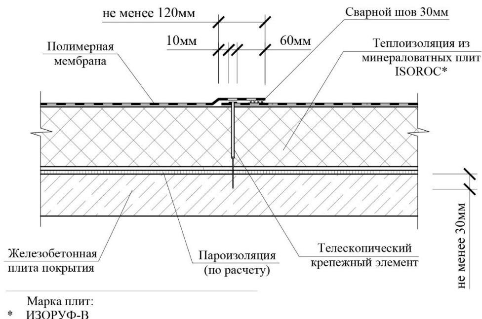
Рис. 13. Устройство гидроизоляционного кровельного ковра из ПФХ-покрытия.
