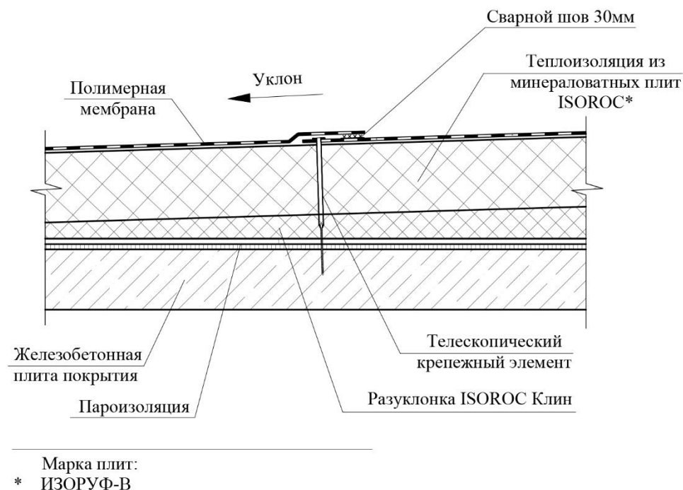
Рис. 15 Устройство гидроизоляционного кровельного ковра из ПВХ-покрытия. «Встречный» шов».
