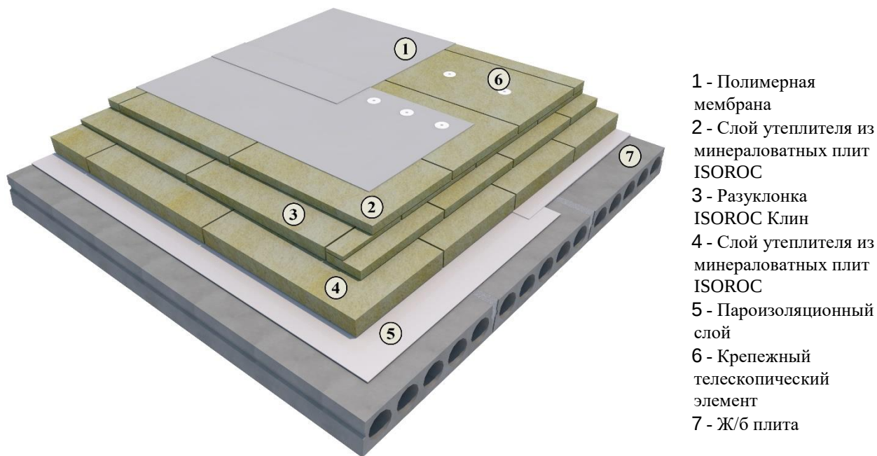
Рис. 1. Конструкция кровельной системы «Изоруф Стандарт ЖБ плита»
