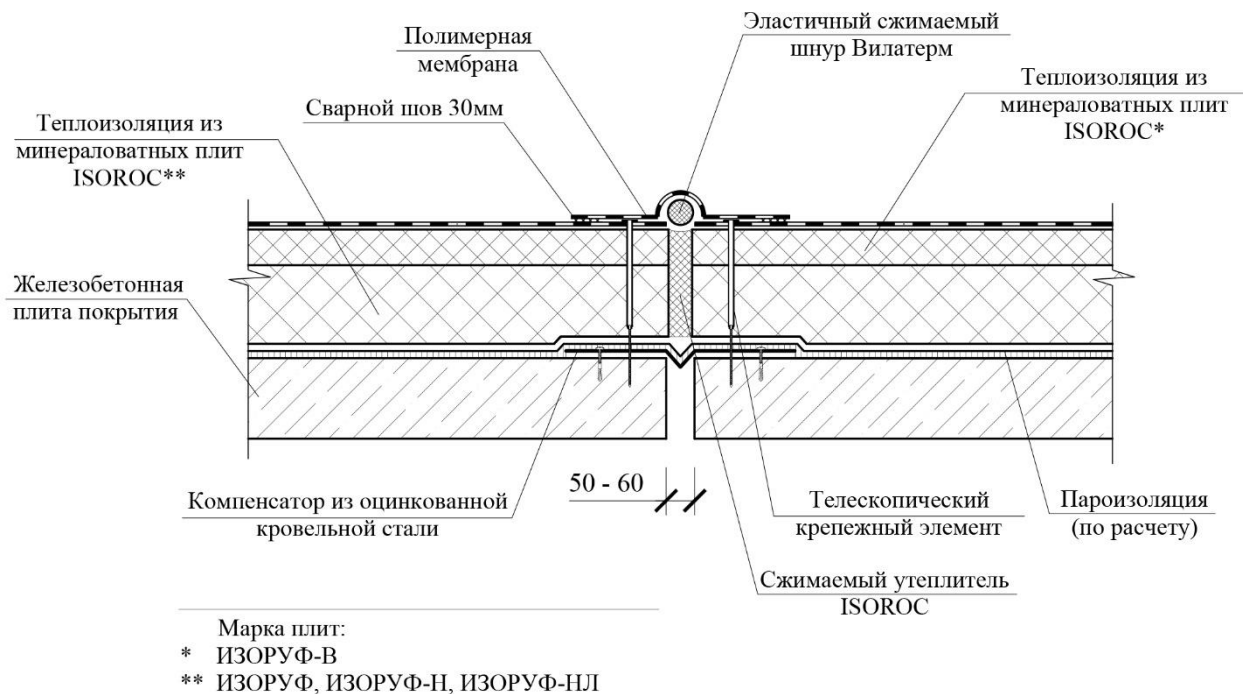
Рис. 33. Деформационный шов Вариант 1.
