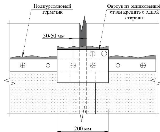
Рис. 27 Краевая рейка на стене из бетонных плит
