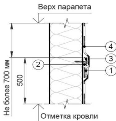
Рис. 30 Примыкание кровли к стене с механическим креплением края кровельного ковра.
