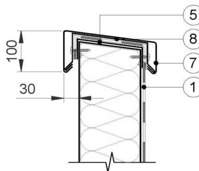
Рис. 29 Примыкание к парапетной стене высотой менее 500 мм с использованием фартука из оцинкованной стали
