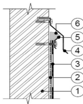
Рис. 23 Примыкание кровли к стене с механическим креплением края кровельного ковра 1– поверхность, выполненная из штучных материалов; 2– геотекстиль термообработанный; 3 – кровельный материал на вертикальной поверхности; 4– отлив из оцинкованной стали; 5– краевая рейка; 6– герметик полиуретановый
