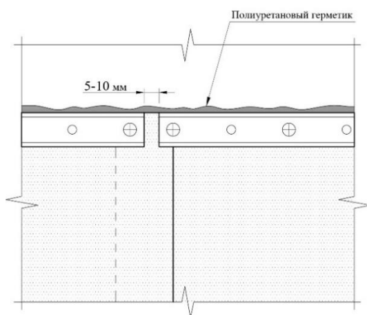
Рис. 24 Зазор между краями соседних реек
