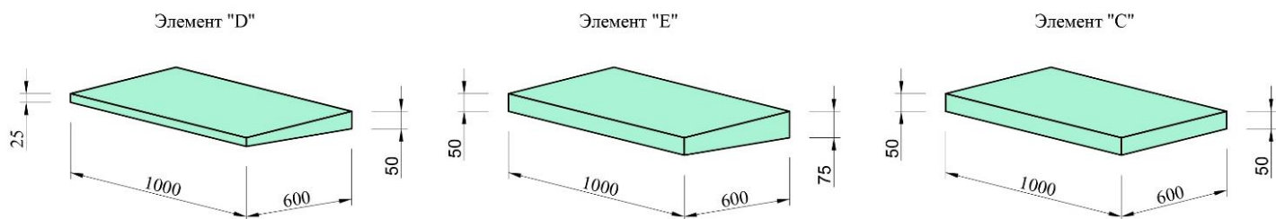
Рис.6. Набор плит ISOROC Клин «D», «Е» 4,2% и добор толщиной 50мм – «С».
