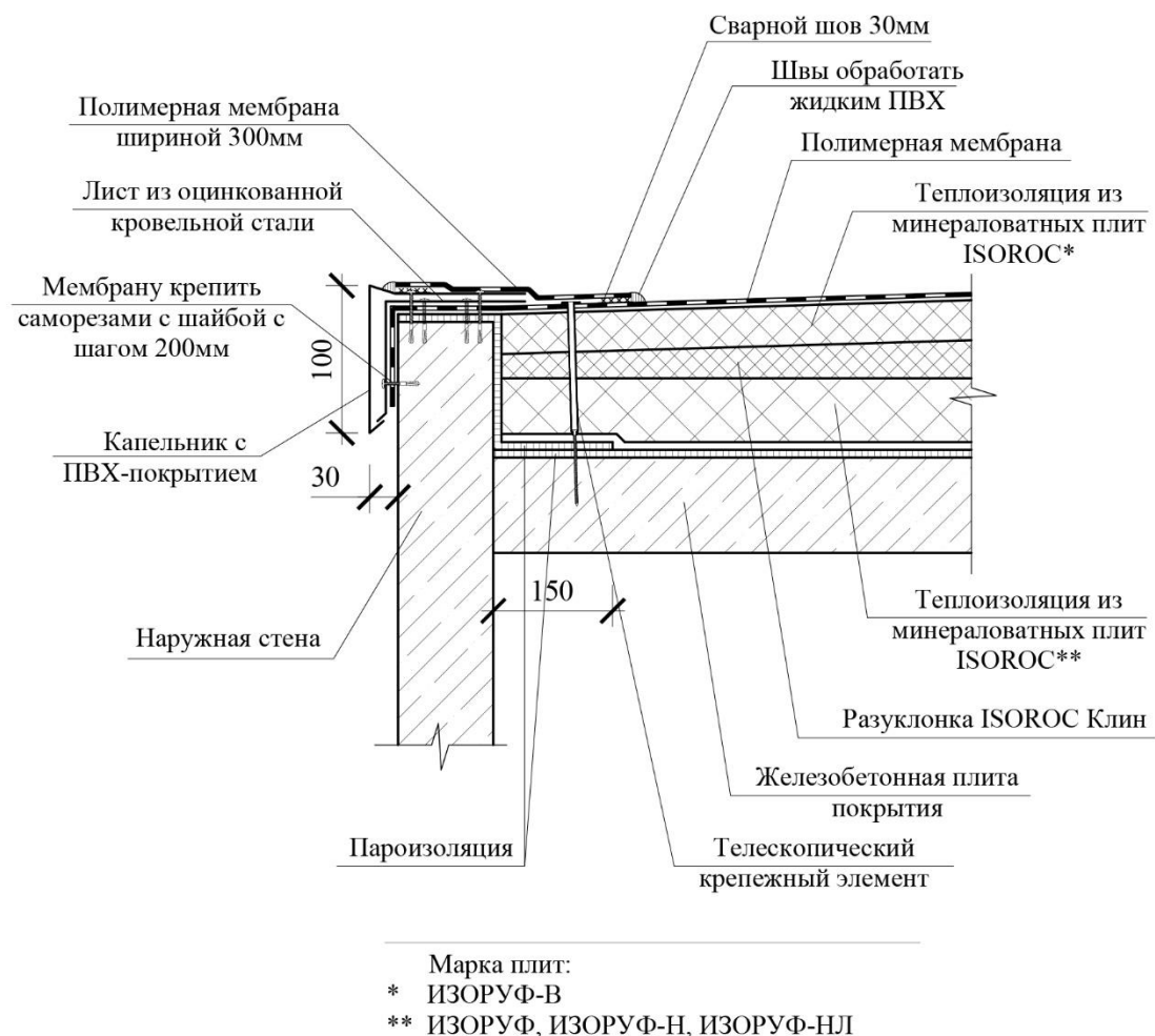
Рис.17 Карнизный свес
