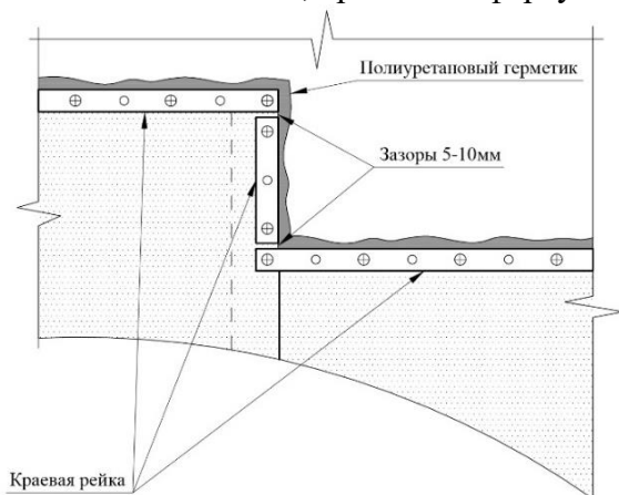
Рис. 26 Обрамление края кровельного ковра краевой рейкой.
