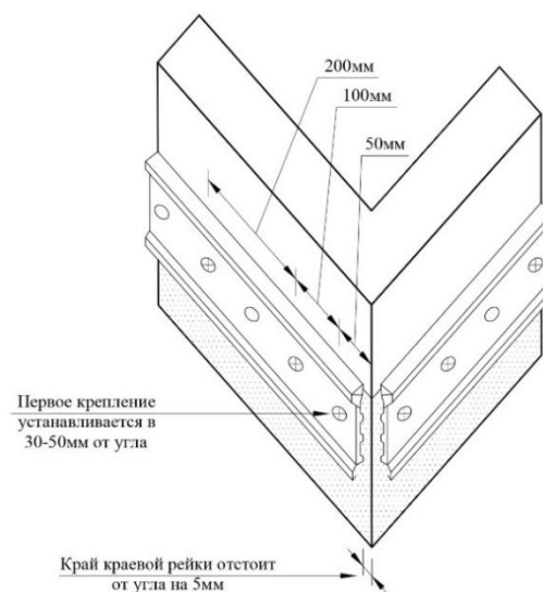
Рис. 25 Установка краевой рейки на углу
